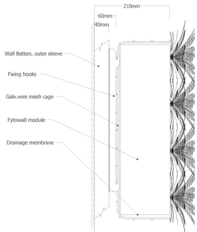
Side Elev.
